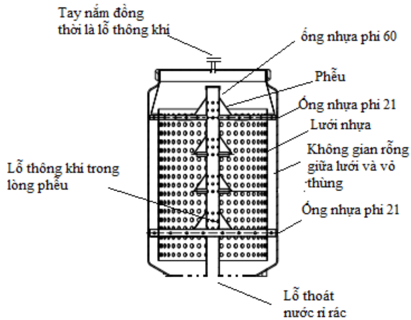
Hình 3: Cấu tạo thùng ủ rác hữu cơ
